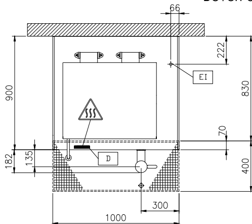
Boven aanzicht
